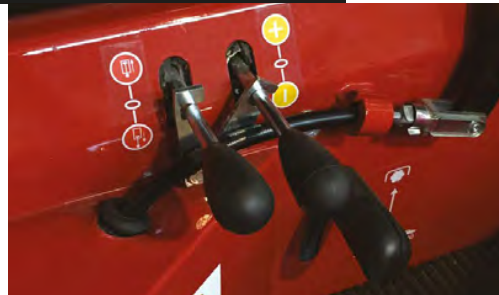
Hydraulischer Verteiler mit 2 Hebeln und 3 Schnellkupplungen hinter dem Sitz. Distributeur hydraulique à 2 leviers avec 3 raccords rapides derrière le siège.
